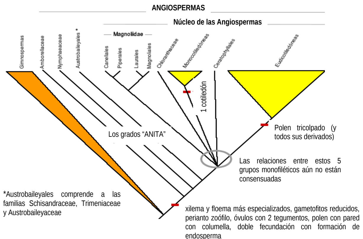
Figura 1. Árbol filogenético dibujado y traducido a partir de APG II (2003), con modificaciones para consensuarlo con Qiu et al. (2005).
