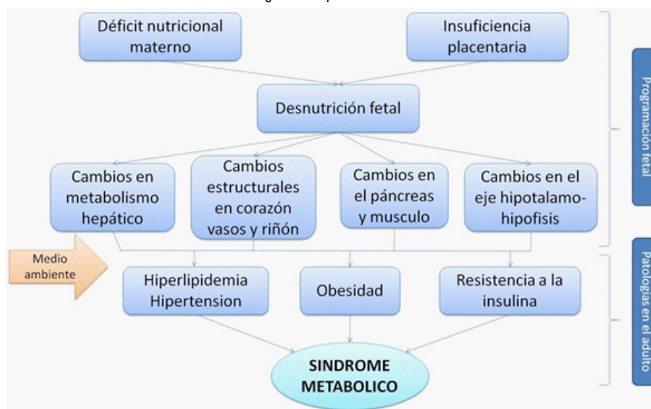
Figura 2. Hipótesis Barker
